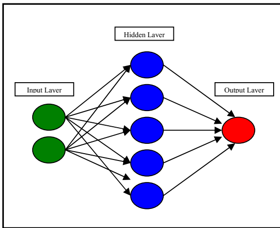
Fig. 6 ANN layers
